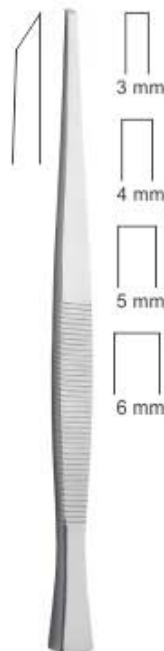
Partsch 170 mm MI-4-504 3mm MI-4-505 4mm MI-4-506 5mm MI-4-507 6mm
